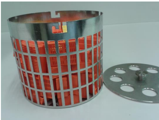
Volle Beladung grosse Kassetten (40 Stück möglich)
