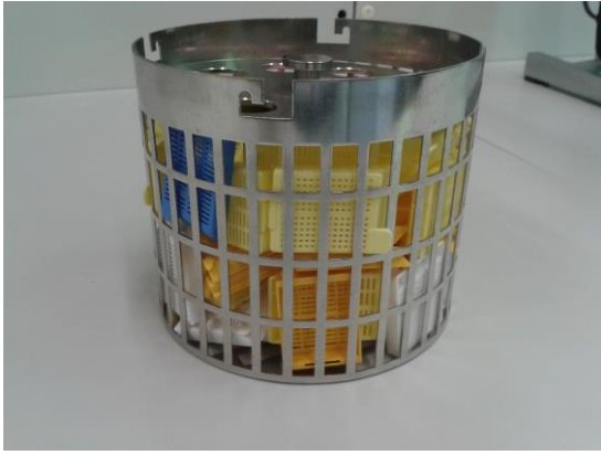
Volle Beladung kleine Kassetten (80 Stück möglich)
